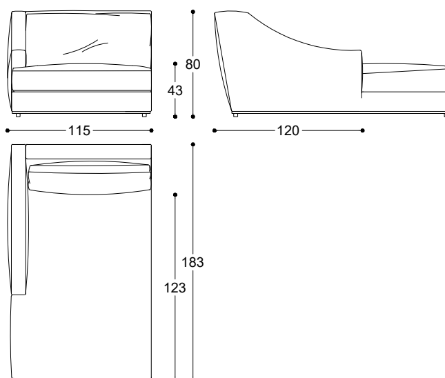
Article: Dormeuse 115 x 183 Left Code: SX-MAR1B Article: Dormeuse 115 x 183 Right Code: DX-MAR1A
